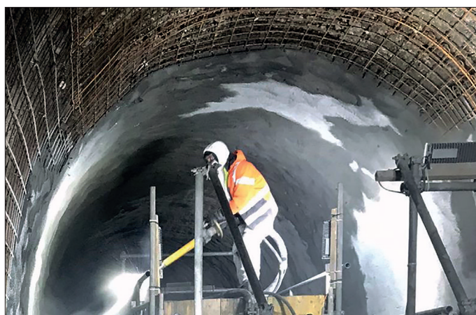
Sicherungsarbeiten im Furka-Scheiteltunnel mit Armierungsnetzen und Spritzbeton Fotos: Ulf Weidle (2)
